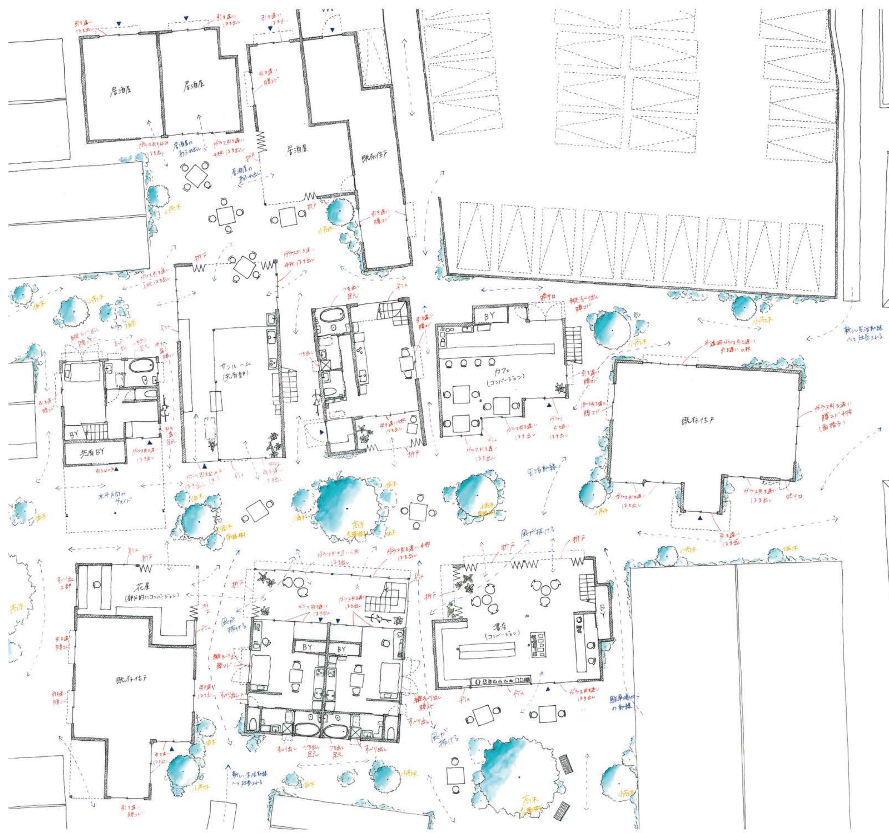
空き地、空き家、既存建築の開口を元に共有環境を構成した平面図 1F スケール 1/150
